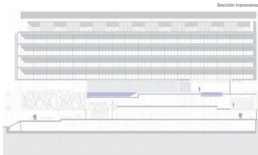
Sección transversal
